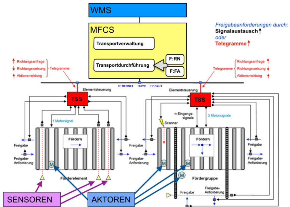
Abbildung 2.5: Neue Funktionskonfiguration (MFC-System ist über TP-RADT mit den Fördererlementen verbunden)
