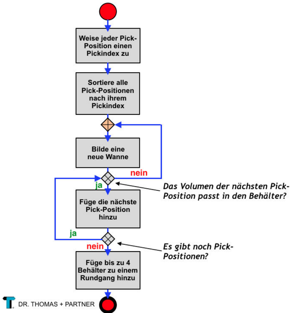
Abbildung 5.14: Ablauf der Wannens-Befüllung und Rundgangsbildung
