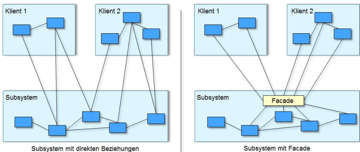
Abbildung 6.13: Subsystem ohne und mit Facade (Gamma, 2004)
