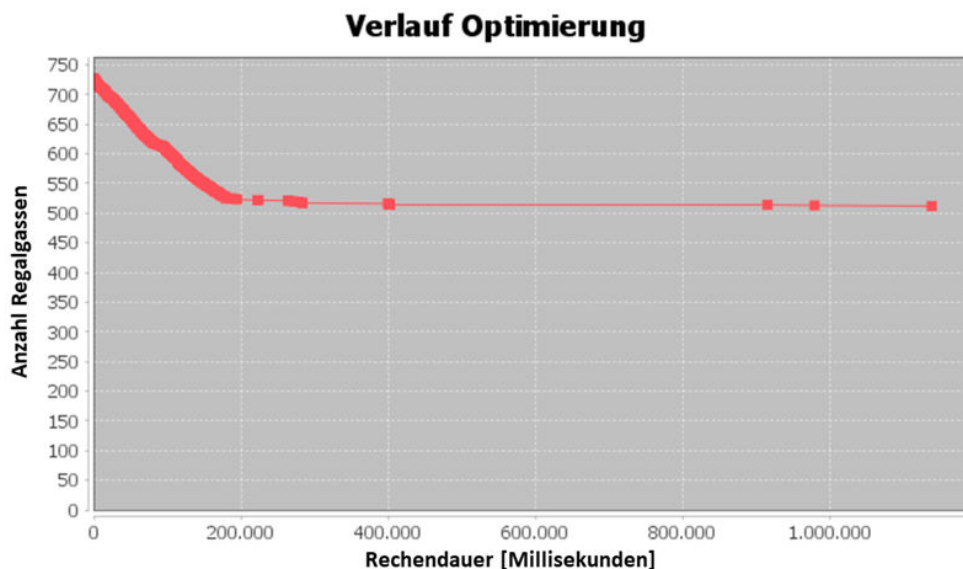
Abbildung 7.4: Verbesserung des Zielfunktionswertes über der Zeit (TUP-Solverlösung)
