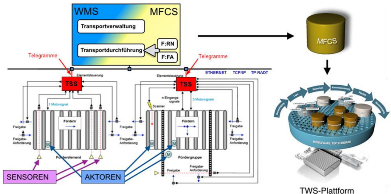
Abbildung 2.8: Komponenten-Architektur adaptiver MFC-Systeme
