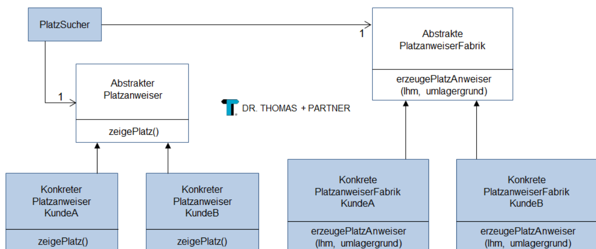
Abbildung 6.10: Abstraktes Fabrik-Muster angewendet auf die Lagerplatzverwaltung
