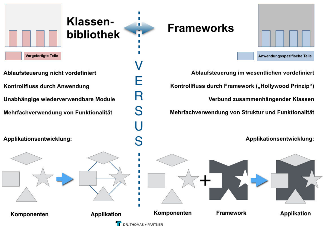
Abbildung 6.12: Klassenbibliothek versus Framework
