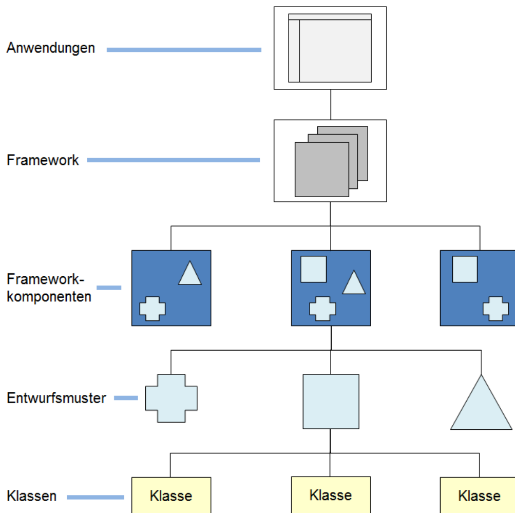
Abbildung 6.11: Komponenten des Frameworks. Struktureller Aufbau / Beziehungen (Johnson 1997)
