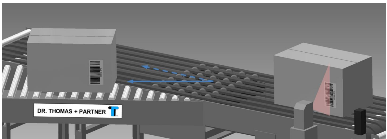
Abbildung 3.8: Stationärer Scanner an Verzweige-Punkt an Fördertechnik
