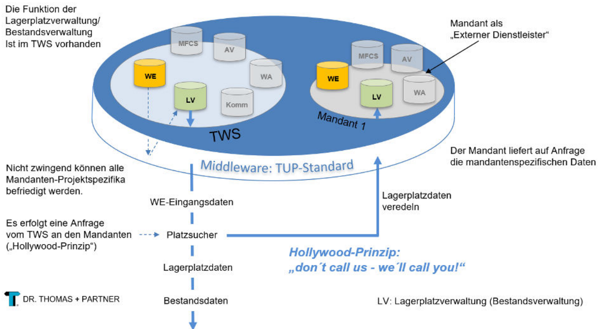
Abbildung 6.19: Hollywood-Prinzip: Lagerplatzverwaltung/Bestandsverwaltung
