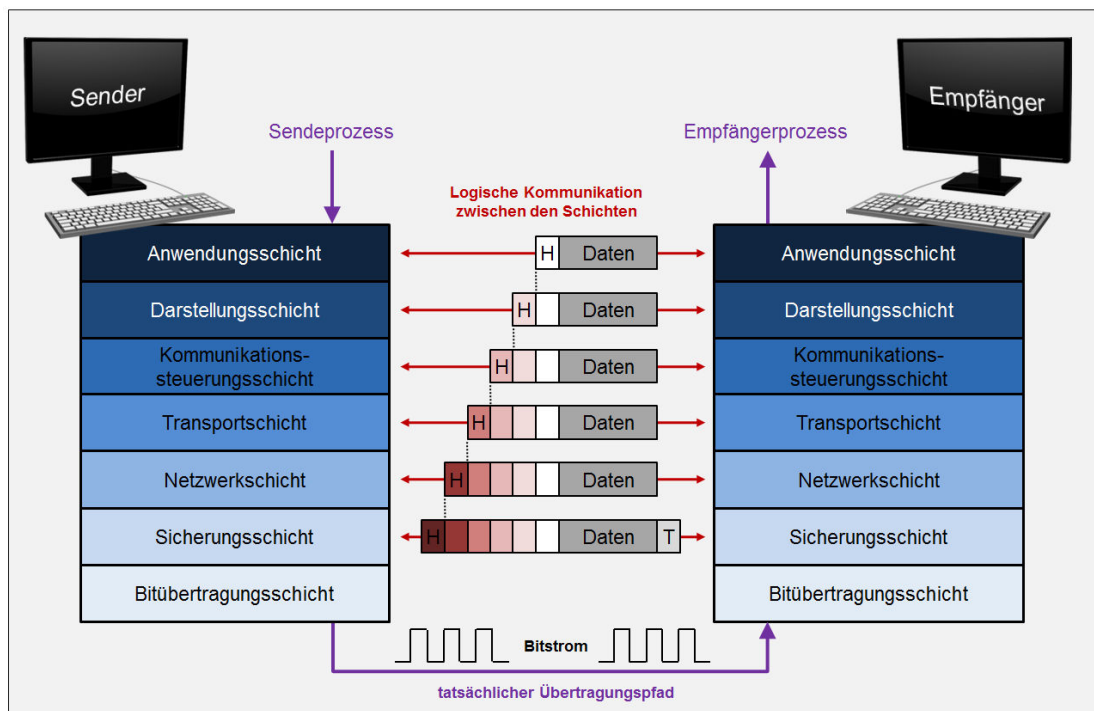
Abbildung 4.4: Das ISO/OSI-Protokoll
