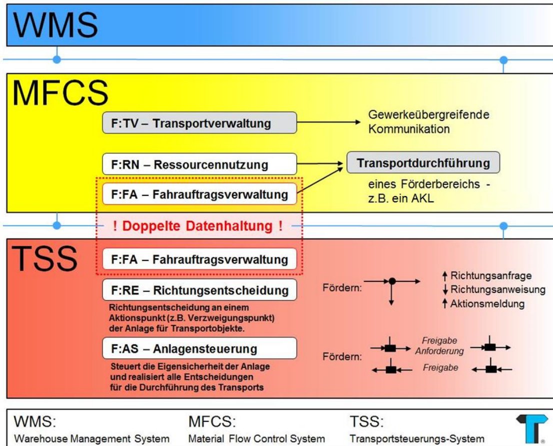
Abbildung 1.4: Klassische Aufgabenzuordnung zwischen dem MFC-System und dem TSS
