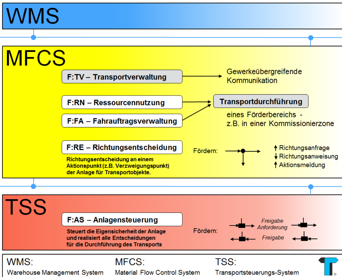
Abbildung 2.2: Neue Aufgabenzuordnung zwischen dem MFCS und dem TSS
