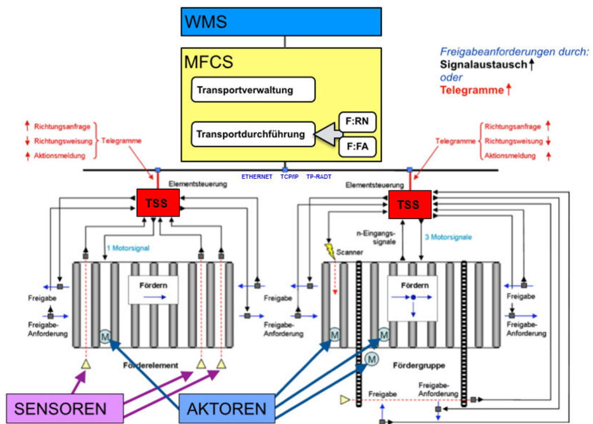
Abbildung 2.5: Neue Funktionskonfiguration (MFCS ist über TP-RADT mit den Fördererelementen verbunden)
